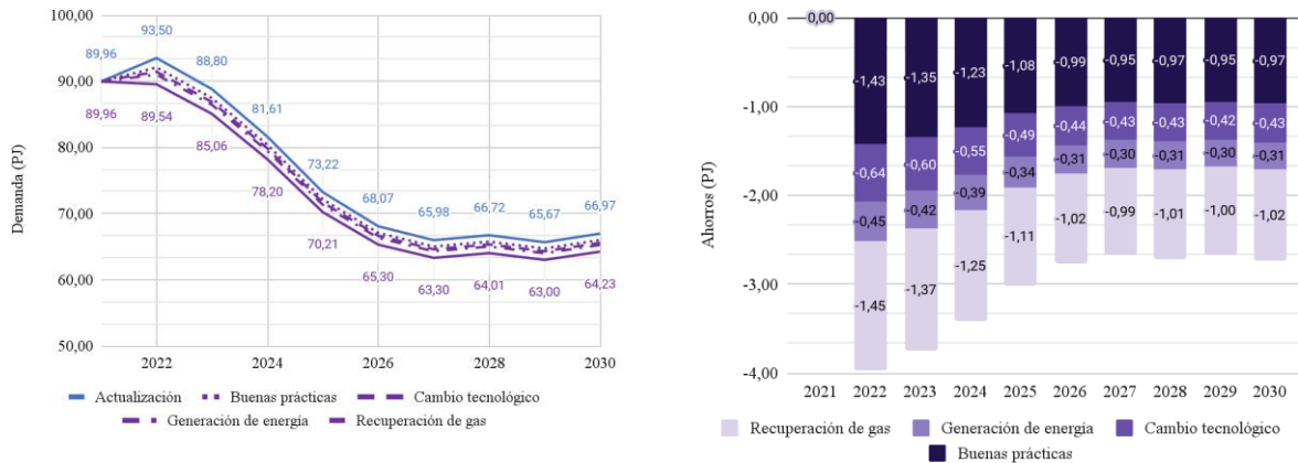
Gráfica 33. Simulación de los ahorros energéticos en el sector de hidrocarburos por la adopción de las medidas analizadas.
